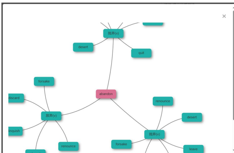
图 4 同义关系
