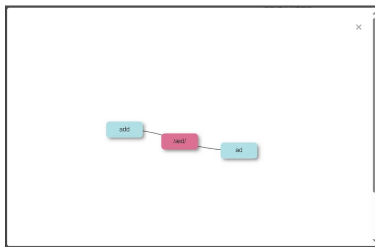
图 6 同音关系
