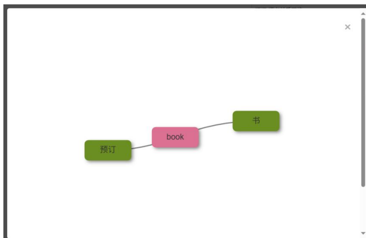
图 5 同形关系
